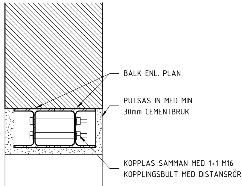
D02 1 : 10
