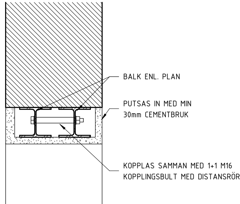
F02 1 : 10
