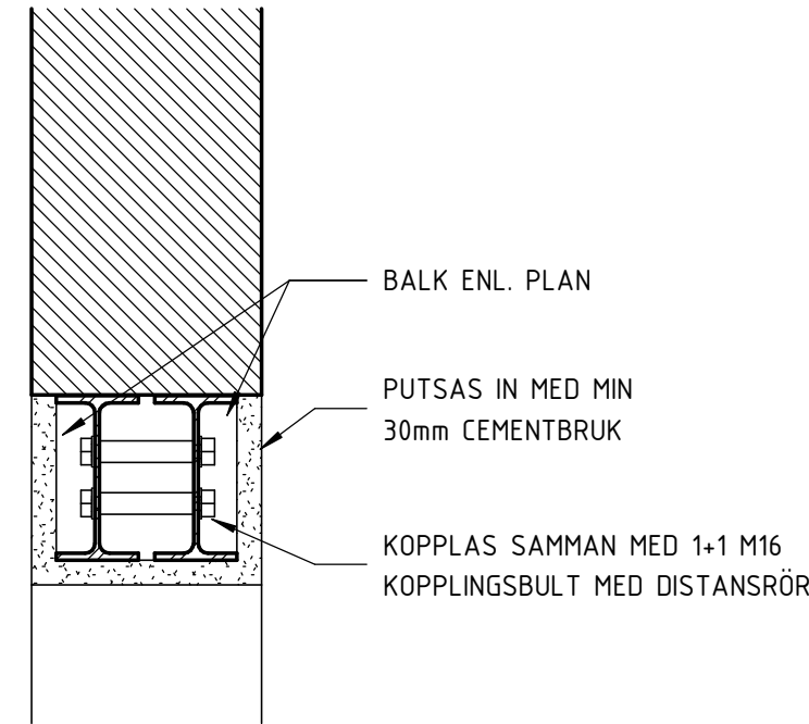
E02 1 : 10
